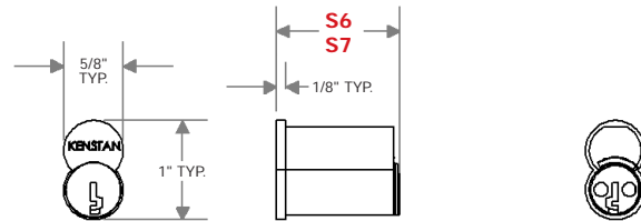
8 keyway core (Patented)
